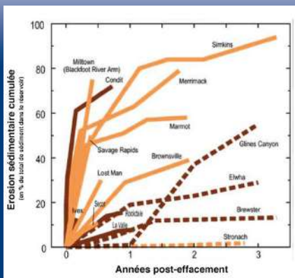
Figure 25. Évolution temporelle de la part de sédiments exportée (en % du volume total de sédiments contenus dans la retenue) après l'effacement du barrage, pour quelques cas documentés aux Etats-Unis.
